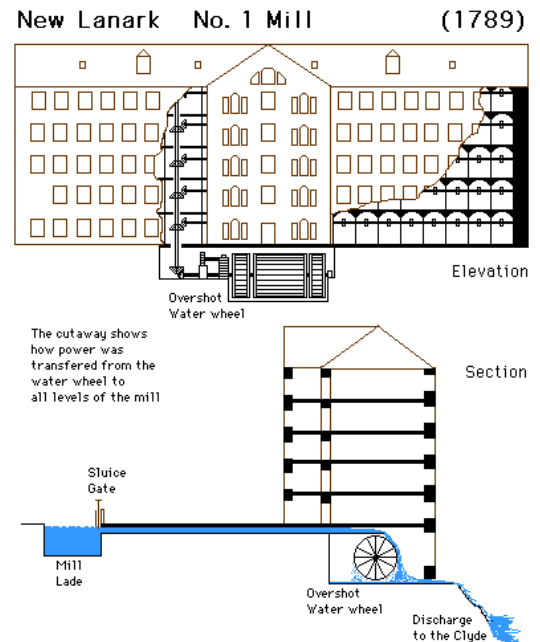
Figura: Dibujo del edificio principal y el mecanismo de utilización de la fuerza motriz del agua, en New Lanark. 64
